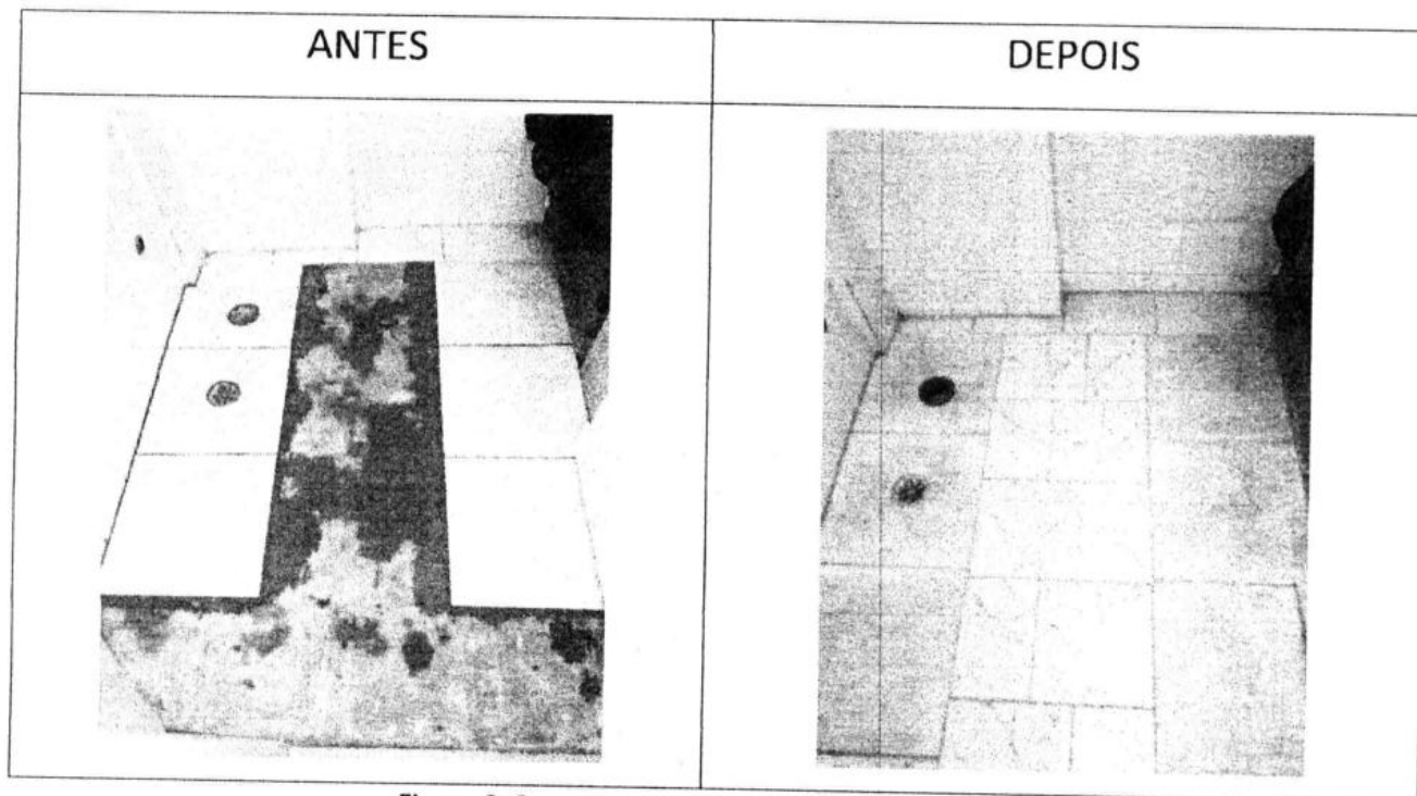
Figura 8: Reparo em cerâmica do piso do sanitário.
